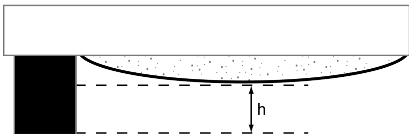
Рис.3 Выпуклый потолок
