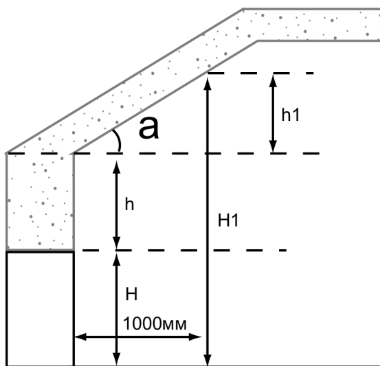
Рис.14 Наклонная притолока
